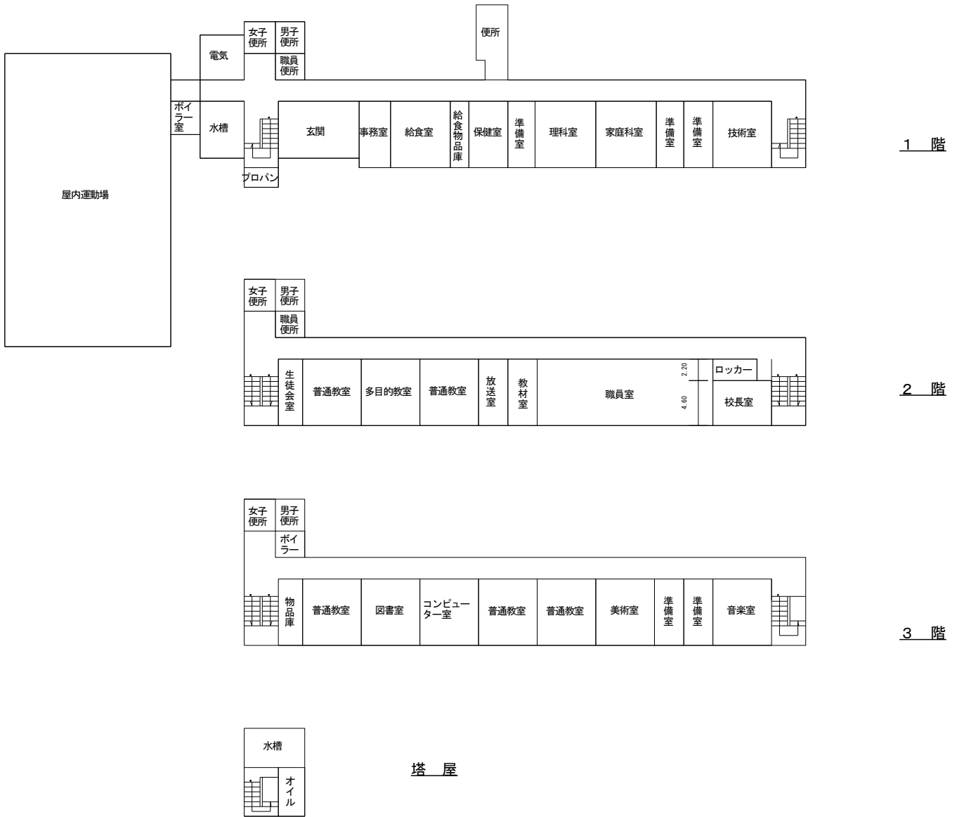
曲淵小中学校 平面図
