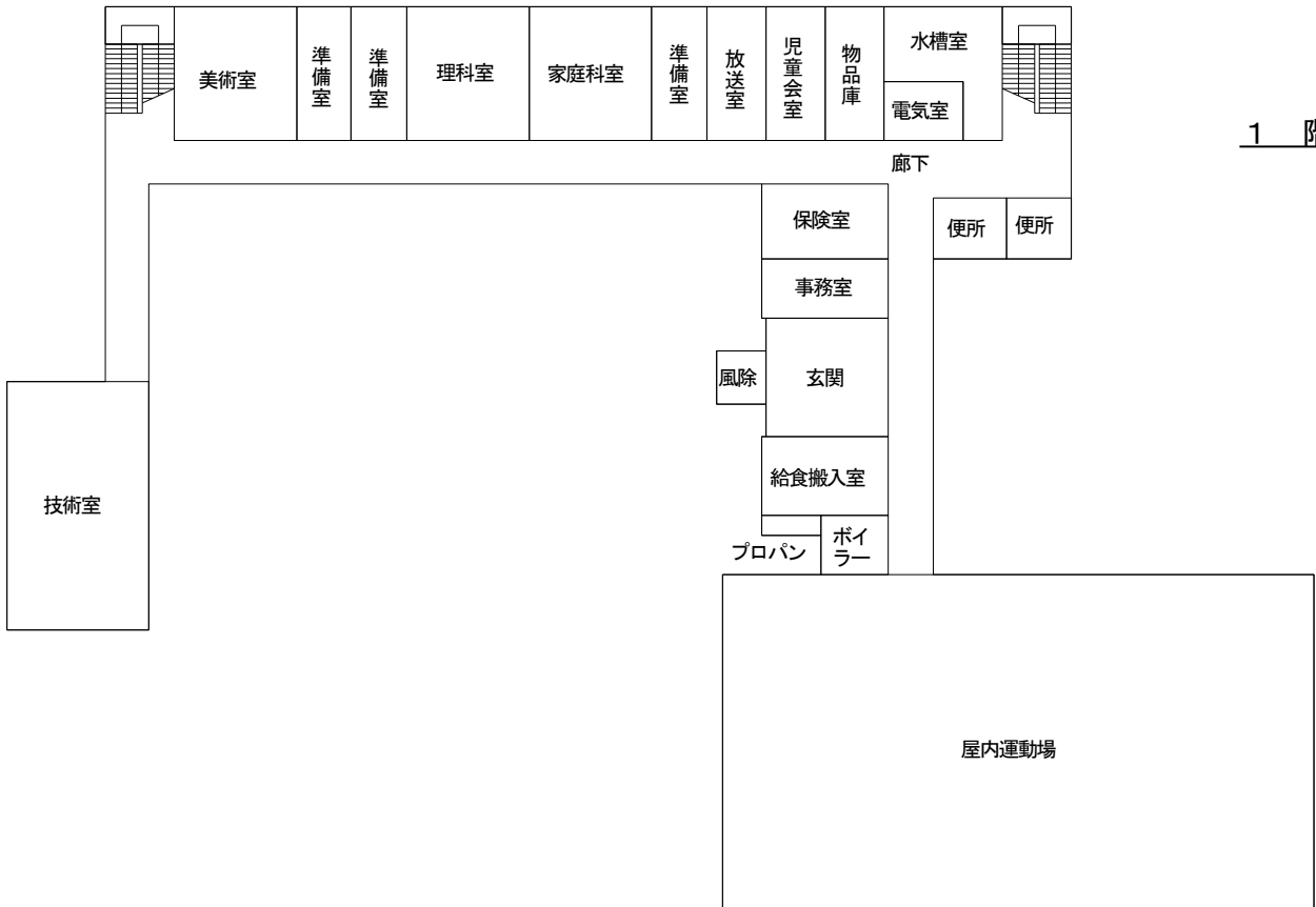
抜海小中学校 平面図
